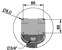
AIW103 Arandela 90°
