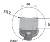
AIWNA /A30 Arandela 30°
